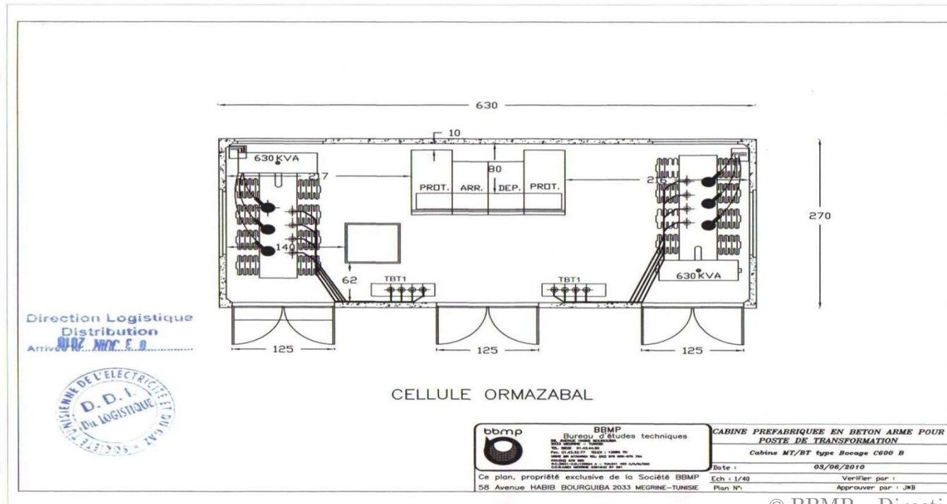
Vue en plan Cabine C 600
